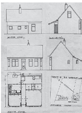
Delen van de bouwtekening hoe het oorspronkelijk was. Tussen de kamer en keuken zijn nog de twee bedsteden.
